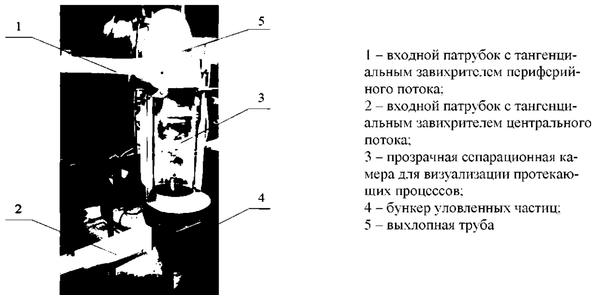
Рис. 1. Лабораторный образец вихревого пылеуловителя с прозрачным цилиндрическим корпусом Fig. 1. Laboratory model of a vortex dust collector with a transparent cylindrical body
