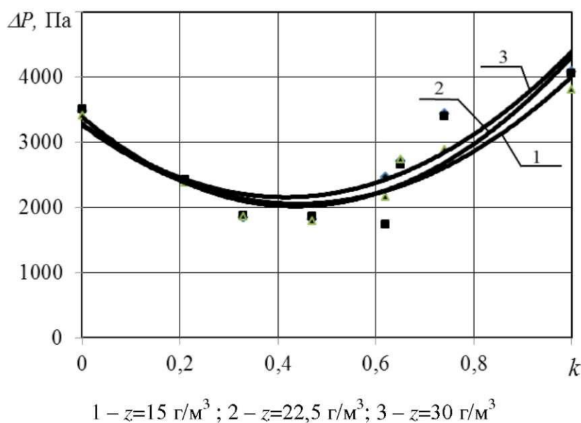
Рис. 3. Зависимости гидравлического сопротивления вихревого пылеуловителя с прозрачным цилиндрическим корпусом от кратности расходов при общем объемном расходе газа Q_0=360 \text{ м}^3/\text{ч} и различных концентрациях мелкодисперсных частиц
